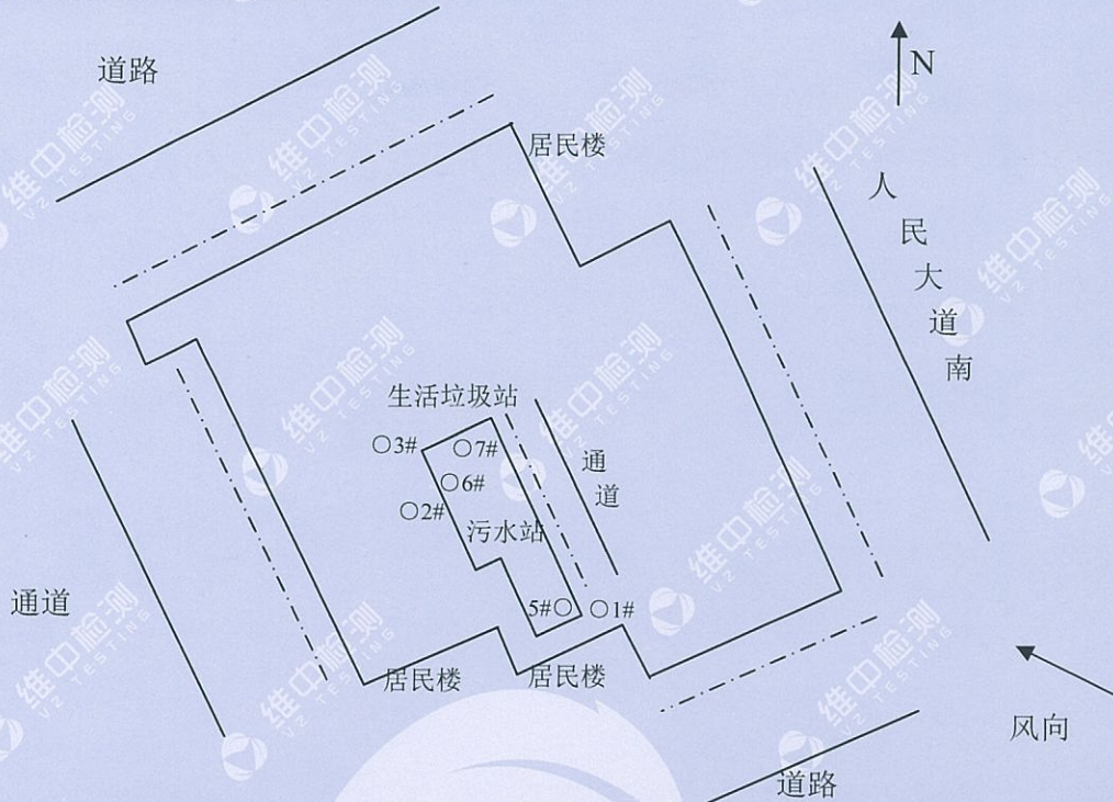
附：无组织废气检测点分布示意图：
